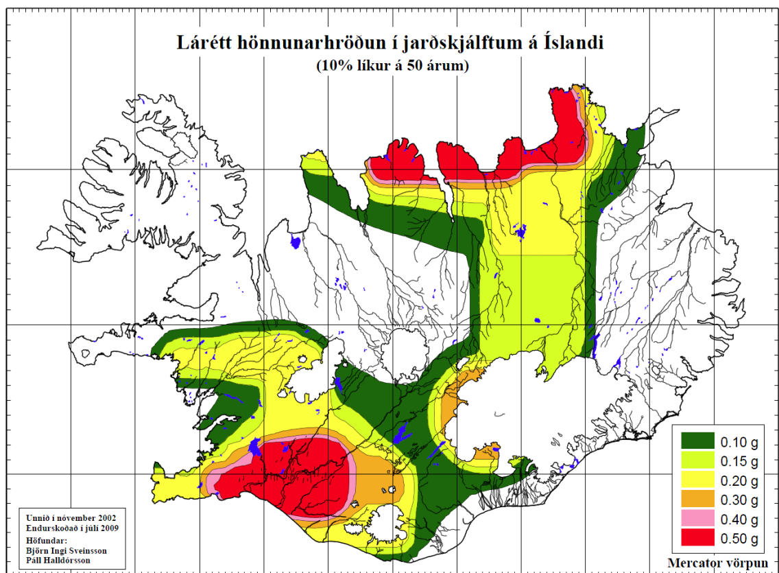
Mynd 13 Skipting Íslands í hönnunarhröðunarsvæði m.v. 500 ára endurkomutíma. Björn Ingi Sveinsson og Páll Halldórsson 2009.
