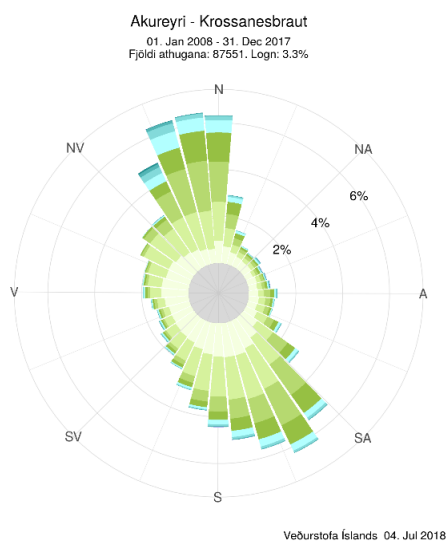
Mynd 12 Vindrósir fyrir Torfur og Krossanesbraut á Akureyri). Veðurstofa Íslands.
