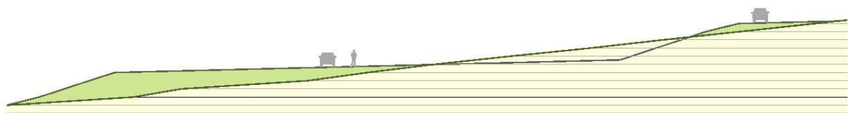
12. mynd. Dæmi um mótun á tjaldflöt með skeringu og fyllingu á núverandi túni.
