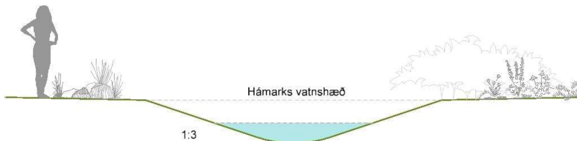
13. mynd. Dæmi um frágang skurða og lækjarfarvega.
